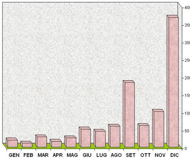
AVVISTAMENTI MENSILI 1978
