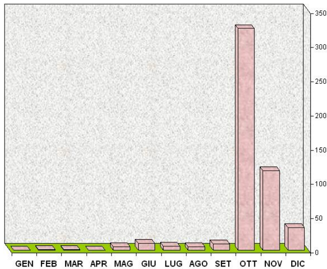
AVVISTAMENTI MENSILI 1954
